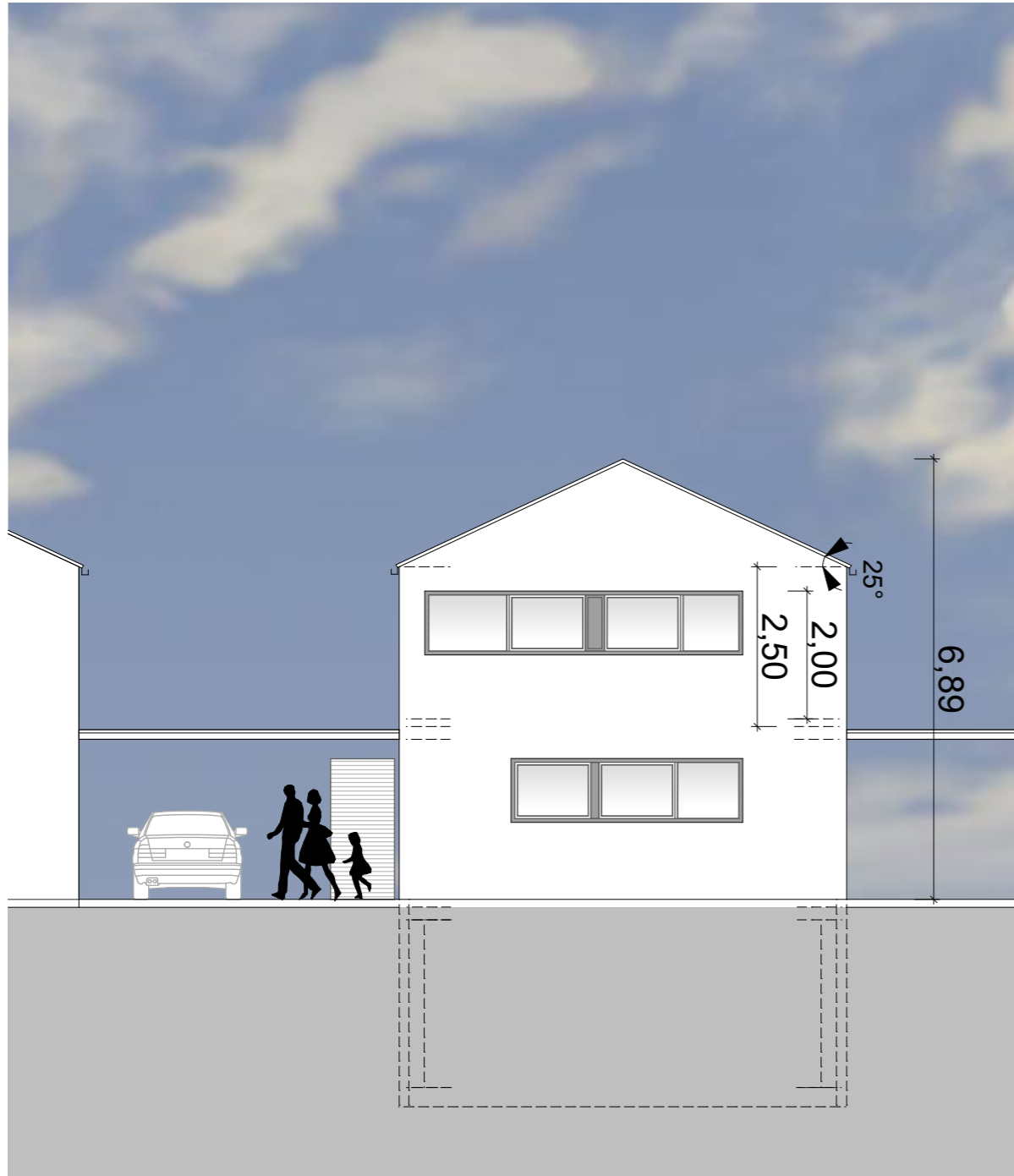
Ansicht Norden
